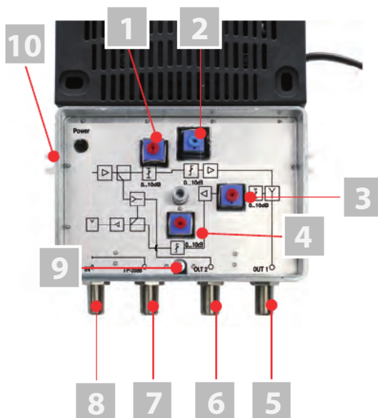
Bild 2: MÜP1 O, Innenansicht
