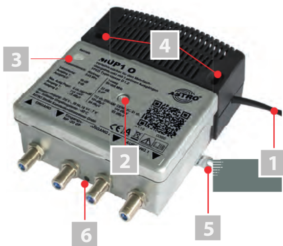
Bild 1: Verteilverstärker MÜP1 O
